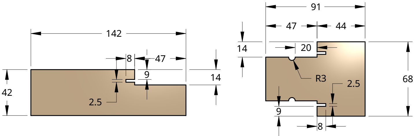
JAMB
